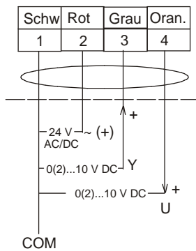
Abbildung 35: Anschluss 0(2) bis 10 V DC
