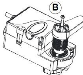
Abbildung 41: Senkrechte Montage des VA9310 auf den Kugelhahn
