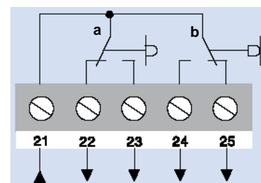
Abbildung 28: Elektrischer Anschluss Hilfsschalter M9108-Axx-5
