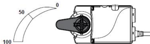
Abbildung 40: Waagrechte Montage des Antriebs VA9310 auf den Kugelhahn
