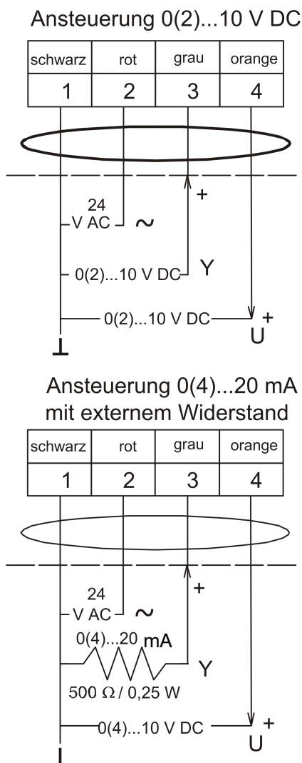
Abbildung 19: Anschluss VA9104-GGA-1S
